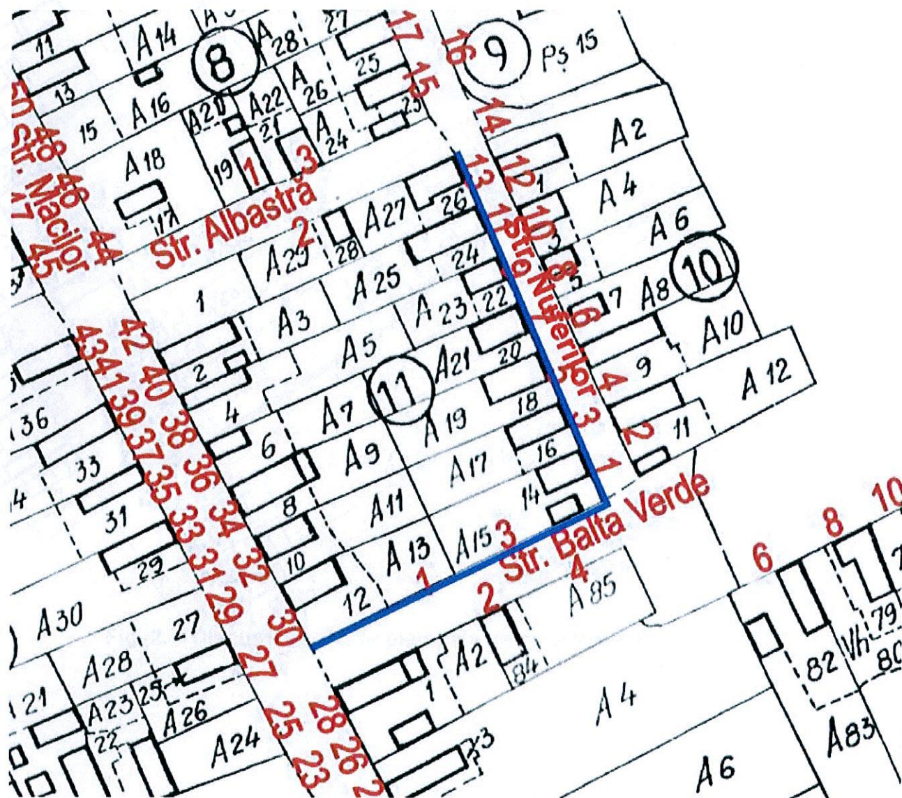
Fig. 1. – Dispunerea aleilor pietonale de pe străzile Nufierilor și Balta Verde
